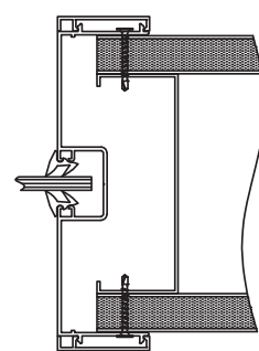
Glass Jamb
