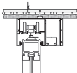
Sliding Door Track
