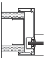
Glass Jamb
